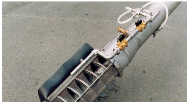
Vista de la cesta del ROTAMAT® Micro Strainer Ro 9
